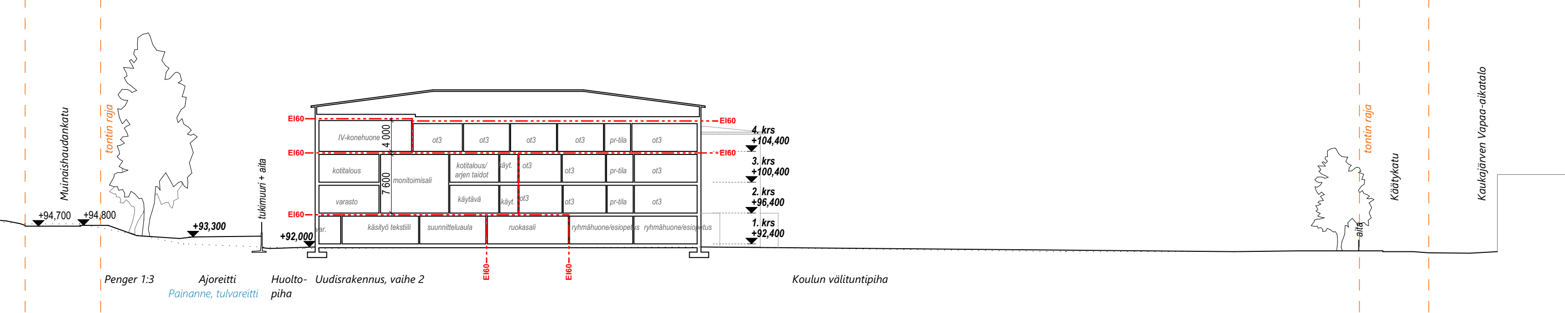
Leikkaus D-D
